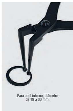
Especialmente projetado para remover e instalar o anel interno no furo profundo.
